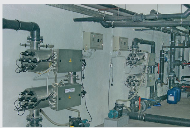
Бассейн, г. Москва, 200 м 3 /ч
